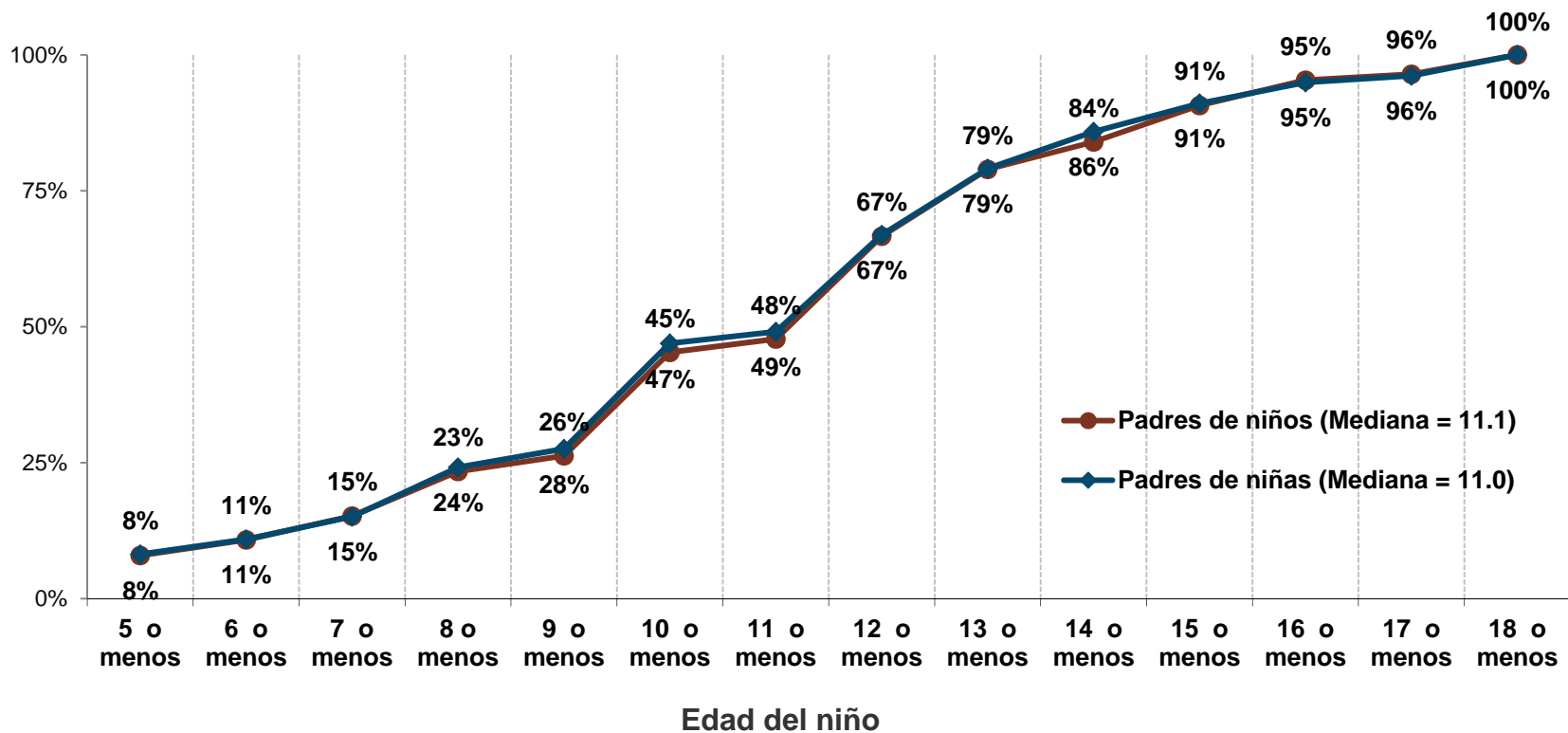
Distribución acumulativa
